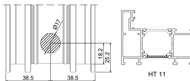
6 - Furação para varões Rods drilling | Perçage pour tiges
