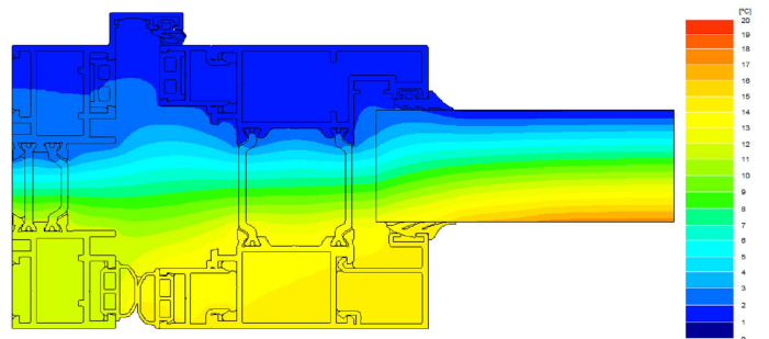
Secção | Section | Section (6a) U_f = 3,10 \text{ W/m}^2\text{K}
