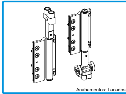
Acabamentos: Lacados 212044 CONJ. DOBR+GUIA INF/SUP HT 8811.1
