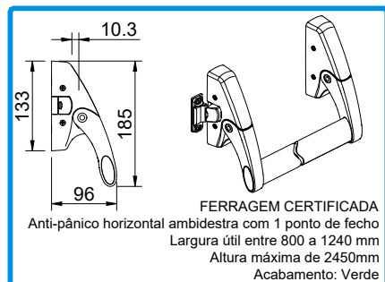
200993 ANTI-PÂNICO HORIZONTAL 6010.1/1200
