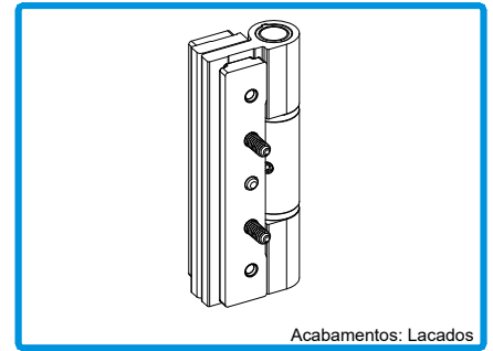
Acabamentos: Lacados 202016 DOBRADIÇA 3 ABAS HT 8815.12
