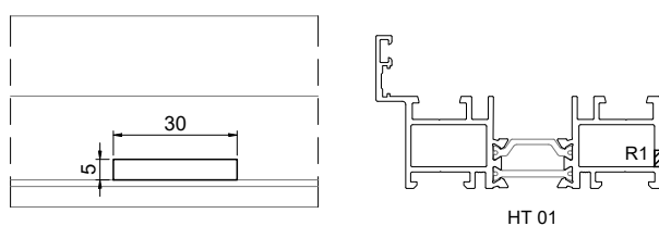
3 - Saída de água Water drainage | Sortie d'eau
