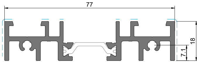
HT 49 Soleira Sill | Seuil
