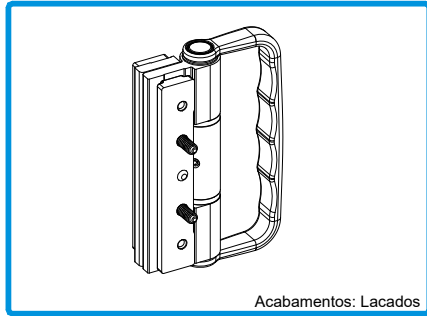
Acabamentos: Lacados 202018 DOBR. 3 ABAS C/ PUX. HT 8816.14
