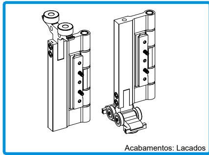
Acabamentos: Lacados 212043 CONJ. DOBR+ROLAMENTO INF/SUP HT 8810.1
