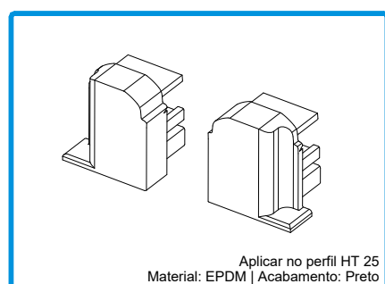
212045 CONJ. TOPOS P/ VD 2126
