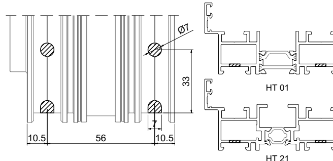
4 - Maquinação para corte de cantos Milling for corners cut | Usinage pour coupe des angles
