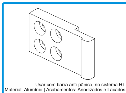
202334 CONTRA-FECHO HT P/ BARRA ANTI-PÂNICO
