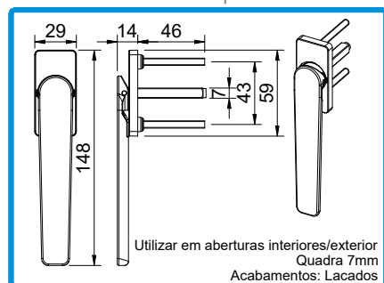
291012 MANÍPULO ARTIC. 3106.30 HT
